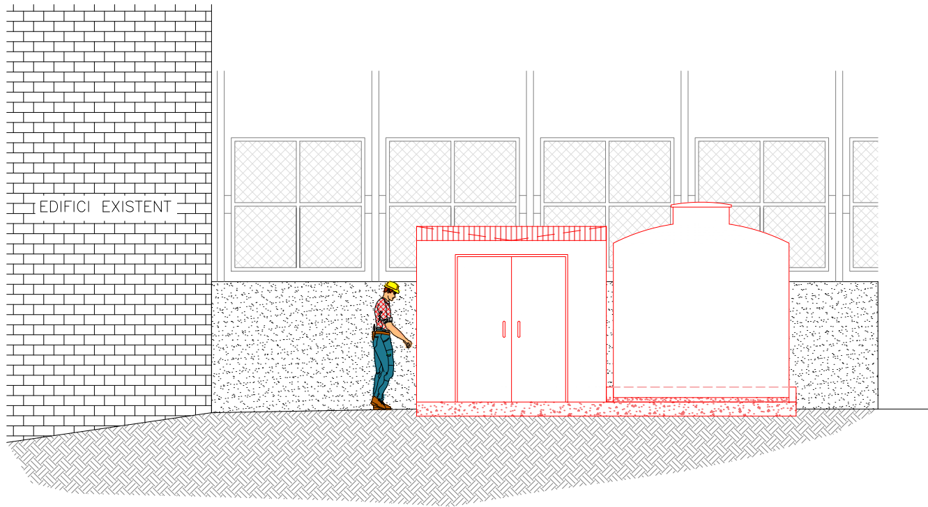
SECCIÓ LONGITUDINAL
