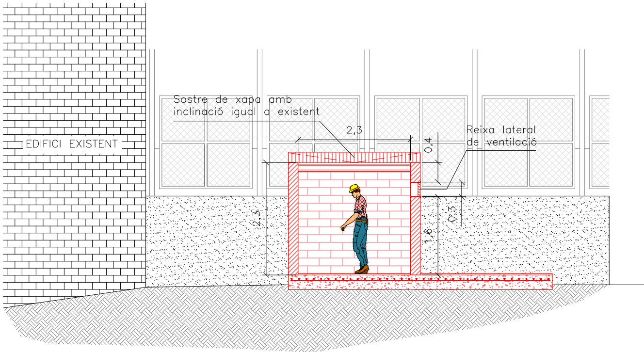
SECCIÓ LONGITUDINAL
