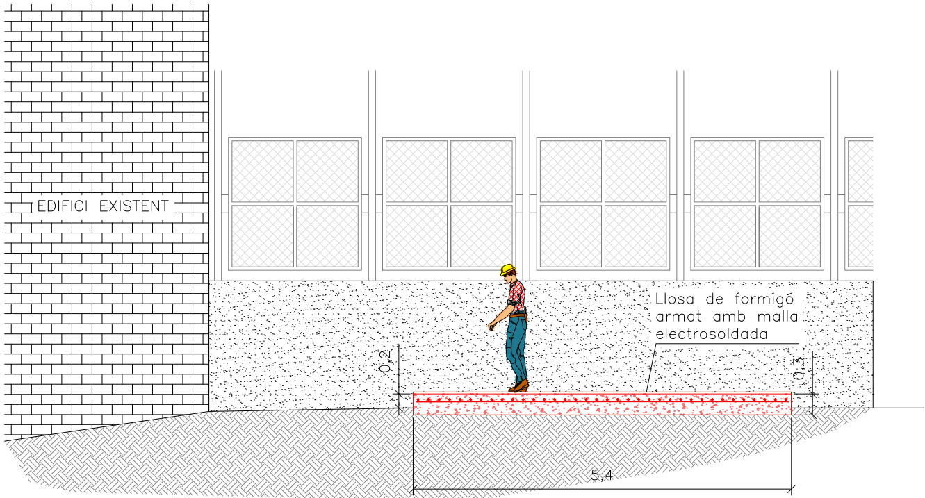
SECCIÓ LONGITUDINAL
