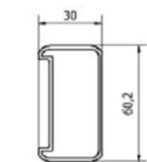
PERFIL VERTICAL
